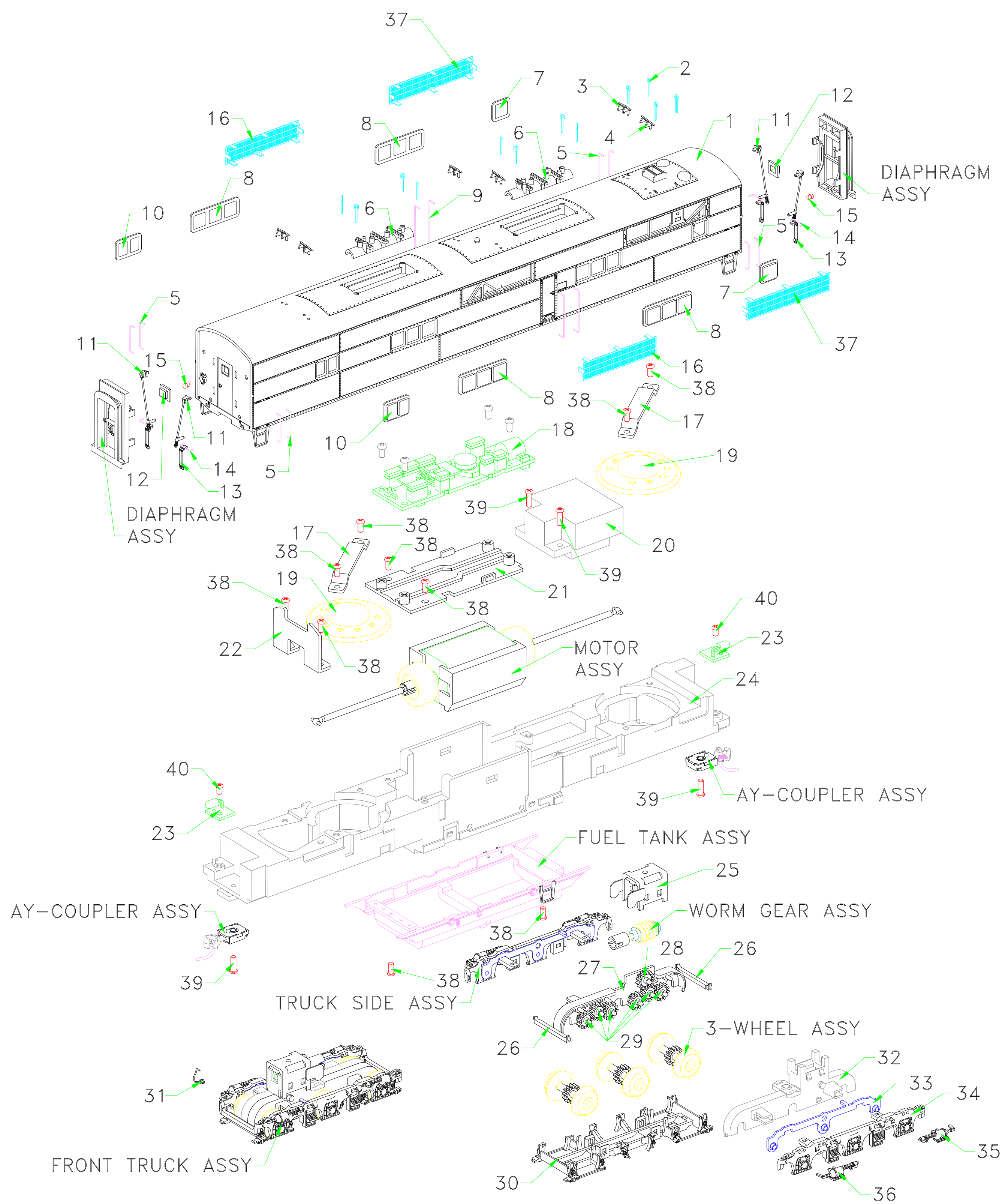
”HO” CD38 ATSF E1 B UNIT(1946/7) EXPLODE TYPE D
